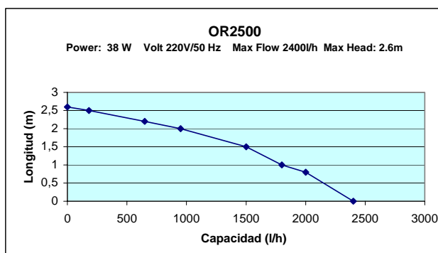
Fig 1: Capacidad de OR 2500, medido sin reducir lado de presión (25 mm, 1")
